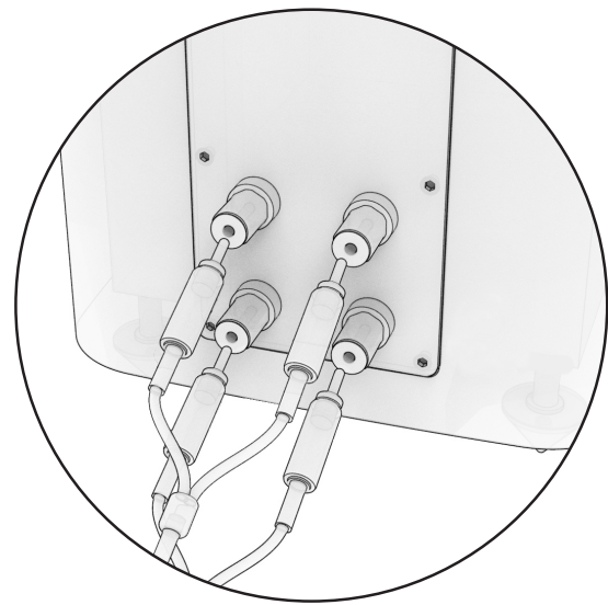
Bi-cablage ou bi-amplification
